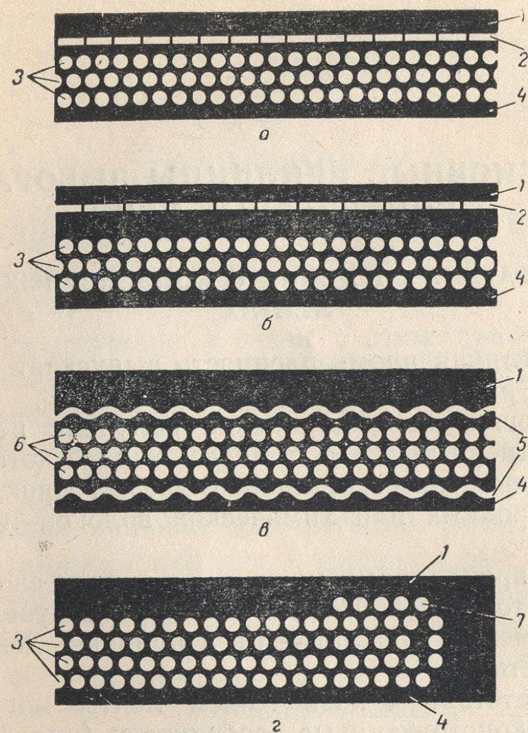
Рис. 1. Конструкции конвейерных лент: 1 — рабочая обкладка; 2 — брекер; 3 — тканевые прокладки; 4 — нерабочая обкладка; 5 — уточная ткань; 6 — основная ткань; 7 — усиленный борт.
