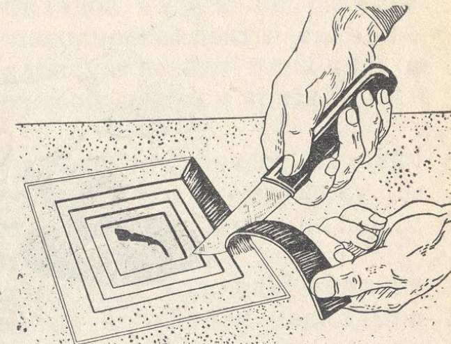
Рис. 37. Срезка обкладочной резины с рабочей стороны ленты.
