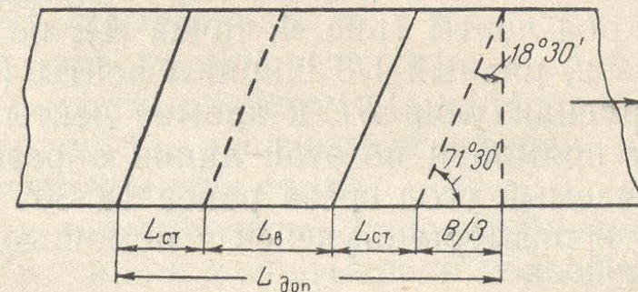
Рис. 6. Схема замены непригодного куска ленты.
