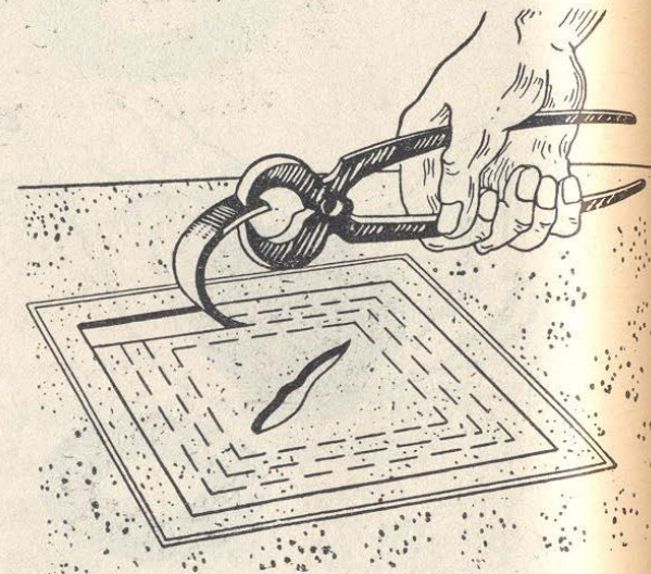
Рис. 35. Разметка ремонтируемого места на ленте, подрезка и отслоение обкладочной резины.
