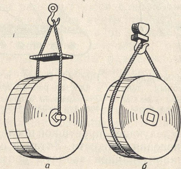
Рис. 43. Переноска рулонов конвейерных лент: а — правильно; б — неправильно.
