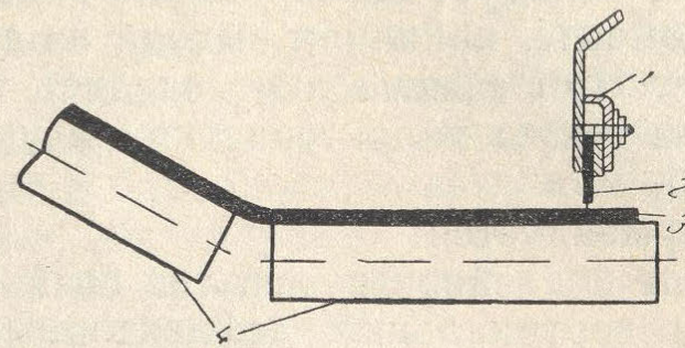
Рис. 29. Установка уплотнений загрузочных устройств:
