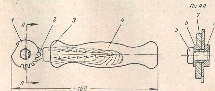
Рис. 45. Резец:
